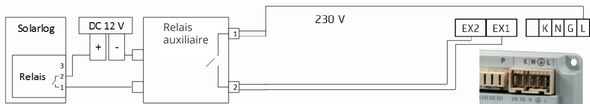
Fig. : Raccordement de la commande au relais auxiliaire
