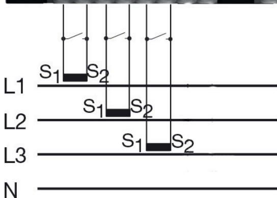
Fig. : Exemple - Schéma de raccordement mesure du courant Utility Meter UMG 104 avec convertisseurs de mesure
