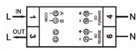
Fig.: Brochage des broches
