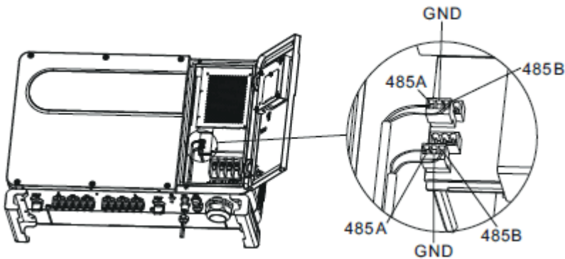
Fig. : Bornier dans l'onduleur
