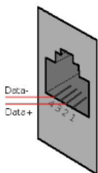
Disposition des broches douille RJ14
