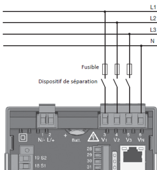
Fig. : Exemple de raccordement pour la mesure de la tension.
