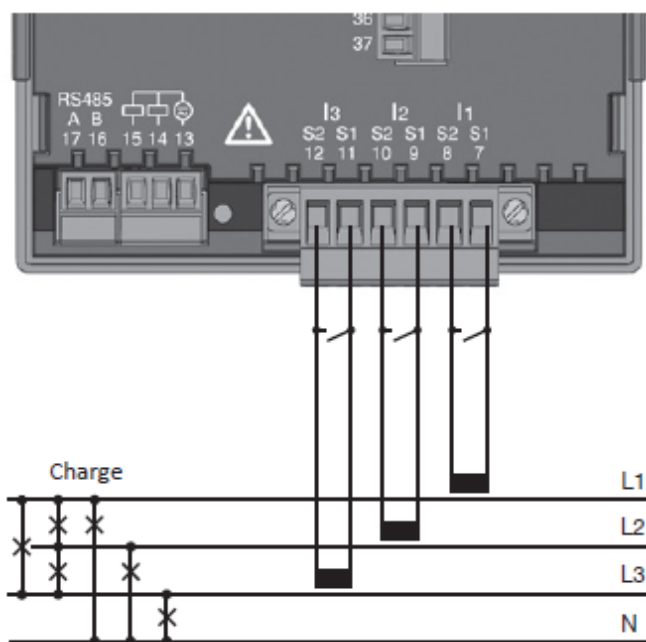
Fig. : Exemple de raccordement „Mesure de l'intensité par transformateur de courant“
