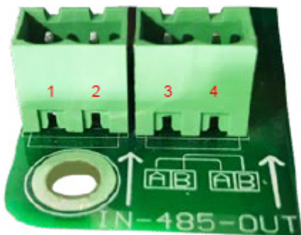
Fig. : Bornier dans l'onduleur (Source : Ginlong)
