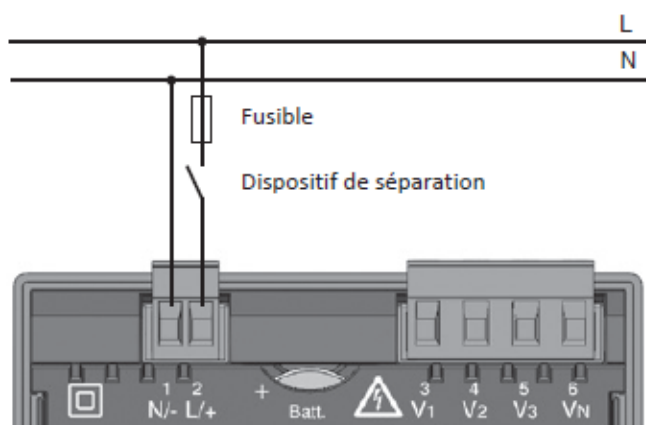
Fig. : Exemple de raccordement „Tension d'alimentation“
