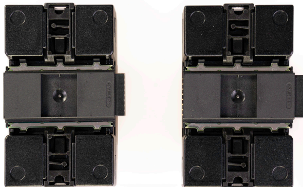
Fig. : Solar-Log Base et Solar-Log MOD 485 avec connecteur de bus.
